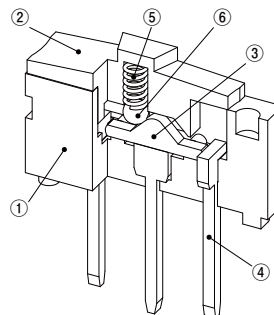
内部構造図 INTERNAL STRUCTURE
